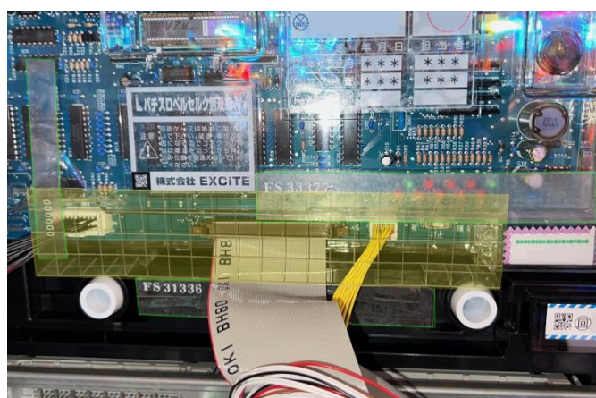
取付け位置
