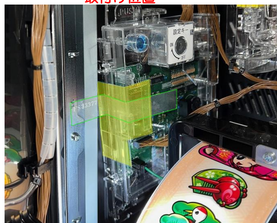
取付け位置
