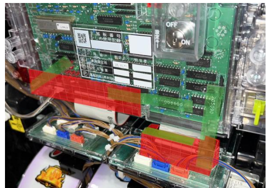
取付け位置
